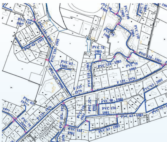
Exemple de plan de réseaux produit par le SDeau50
